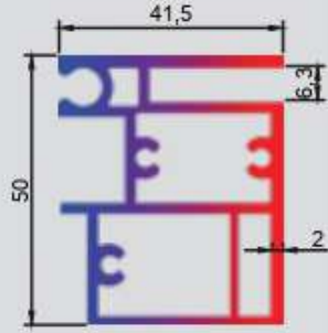
T. 2374 - 1.847 kg/m Hareketli Dikme / Yatay
