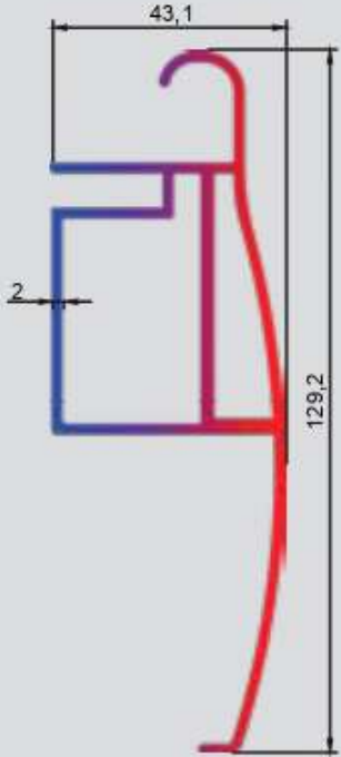
T. 2373 - 1.847 kg/m Hareketli Küpeşte
