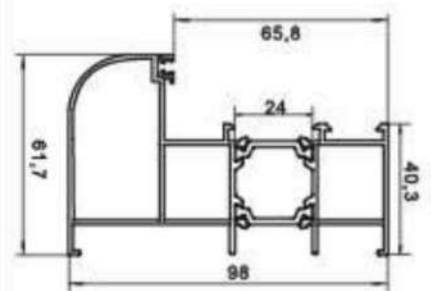
Štok balon 100 mm
