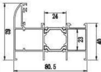
Štok balon 80 mm
