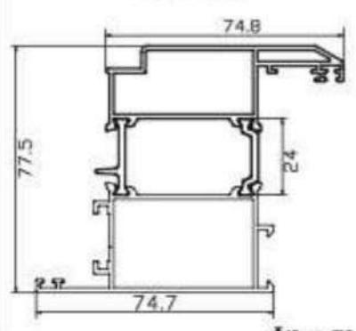
Krilo vrata
