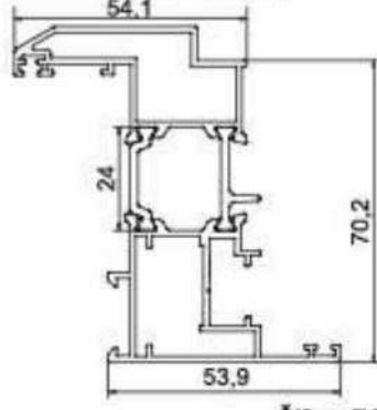
Krilo multilock
