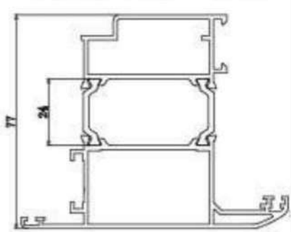
Krilo vrata spoljno otvaranje
