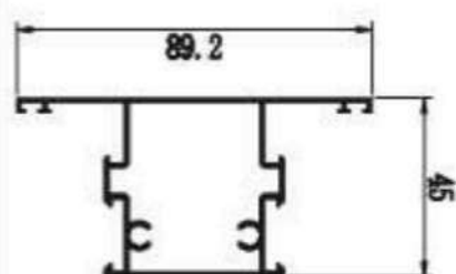
Te prečka
