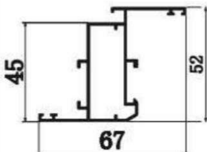
Kriilo prozora
