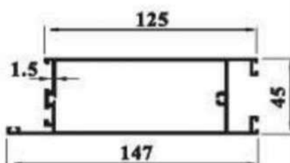
Parapet
