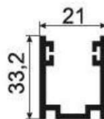
Aluminijumska vođica za rolokomarnik
