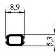
NO : 2345 AGIRLIK : 0.055 kg/m
