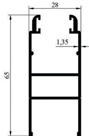
NO : 2336 AGIRLIK : 0.759 kg/m
